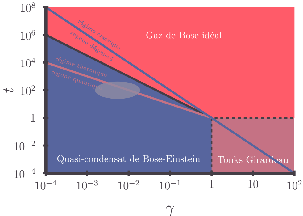
FIGURE II.4 – Diagramme des régimes principaux du gaz de Lieb–Liniger : gaz de Bose idéal, TG et qBEC , en fonction des paramètres adimensionnés \gamma et t . Les courbes noires, bleues et orange délimitent les cross-overs entre régimes. La zone grise correspond aux paramètres expérimentaux explorés pendant la thèse. Figure adaptée de [BDW11].
